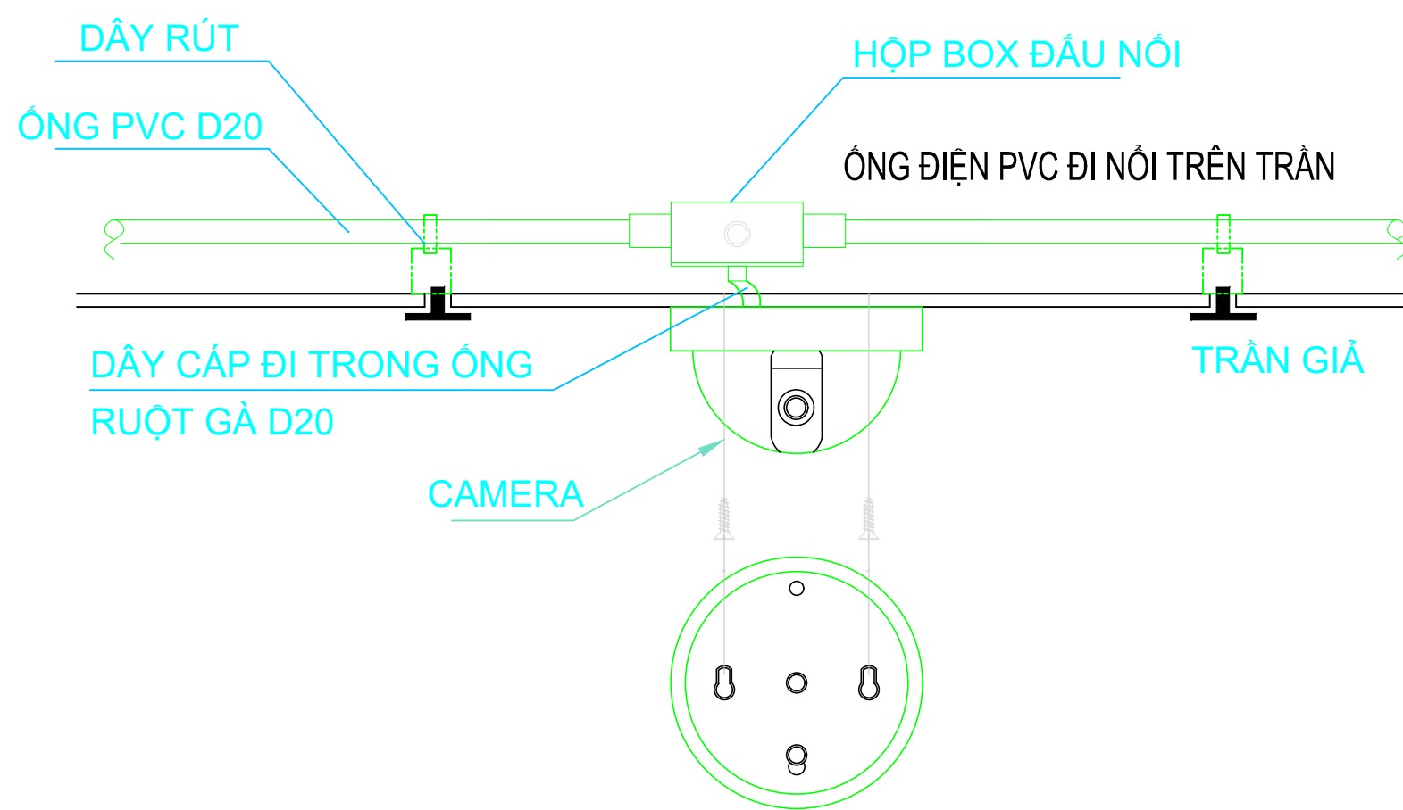
CHI TIẾT LẮP ĐẶT CAMERA DOME
