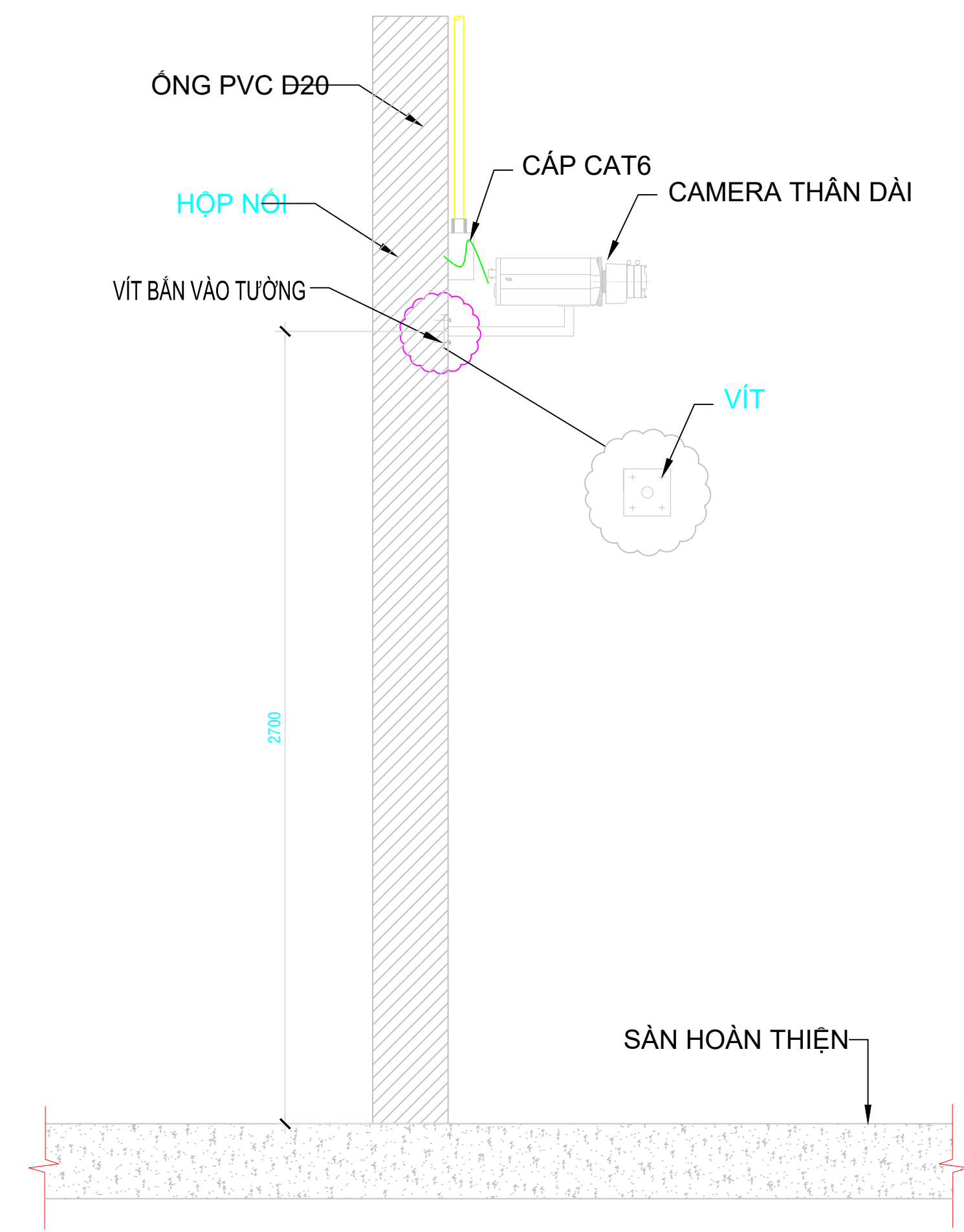
CHI TIẾT LẮP ĐẶT CAMERA THÂN DÀI GẮN TƯỜNG
